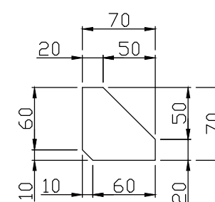
PEÇA G CHAPA # 1/8" QUANTIDADE : 16 PÇS
