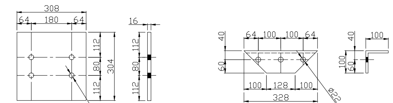
PEÇA E CANTONEIRA L 4" # 3/8" QUANTIDADE : 02 PÇS
