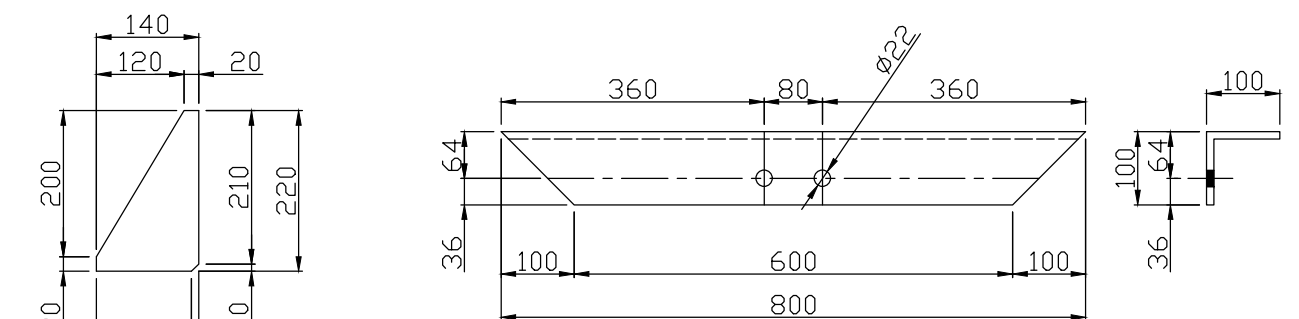
PEÇA F CANTONEIRA L 4" # 3/8" QUANTIDADE : 02 PÇS
